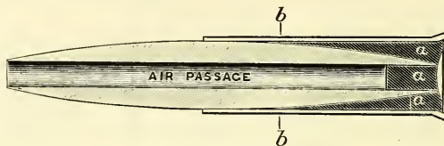
Hebler Krnka Tubular Bullet.
